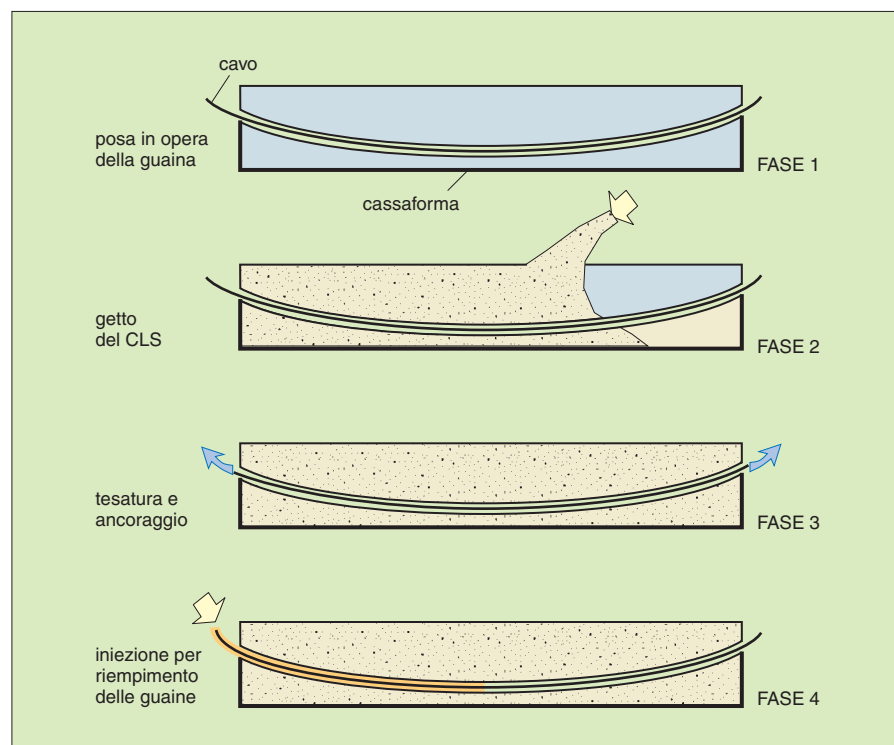
FIGURA 8 Sistema di post-tensione (precompressione a fili scorrevoli).
